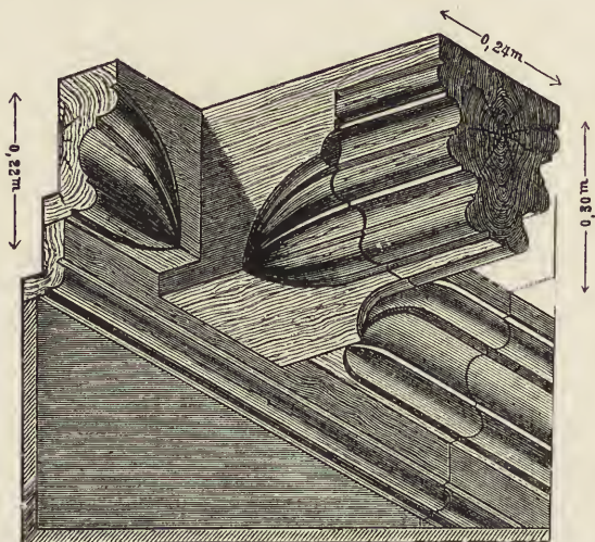
Fig. 46. Ehrenberg, Balkendecke.
